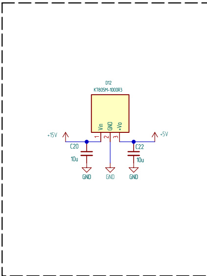
Питание +5В
