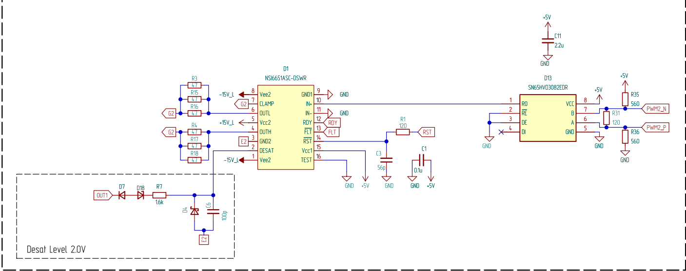
Питание +5В
