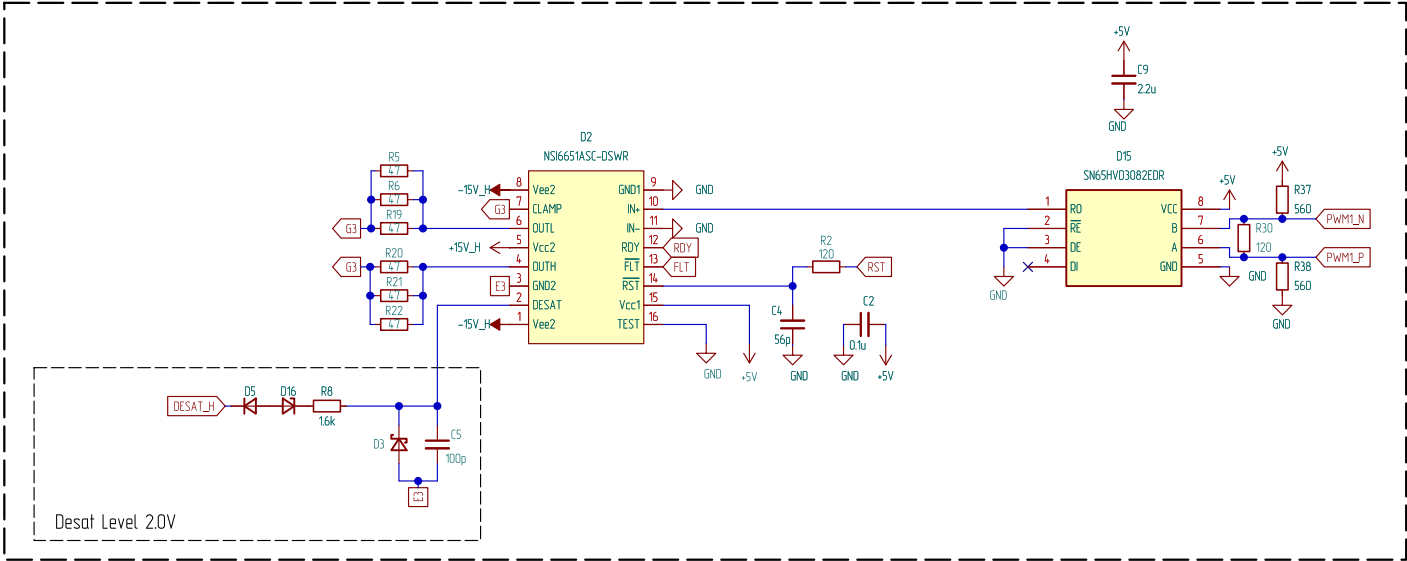
Драйвер нижнего ключа
