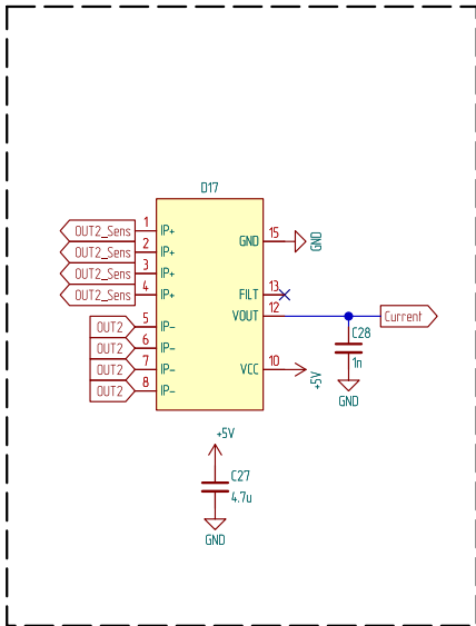
Датчик тока
