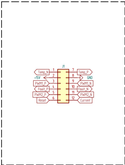
Управляющий разъем
