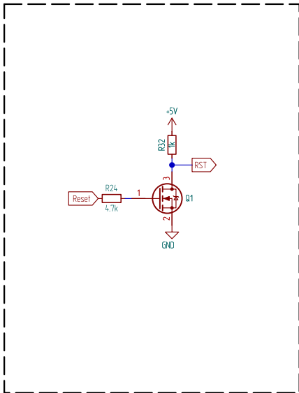
Сброс ошибки драйвера
