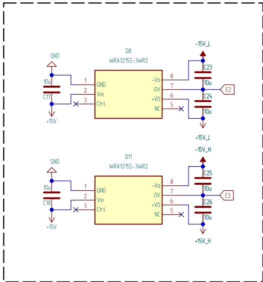
Питание драйверов
